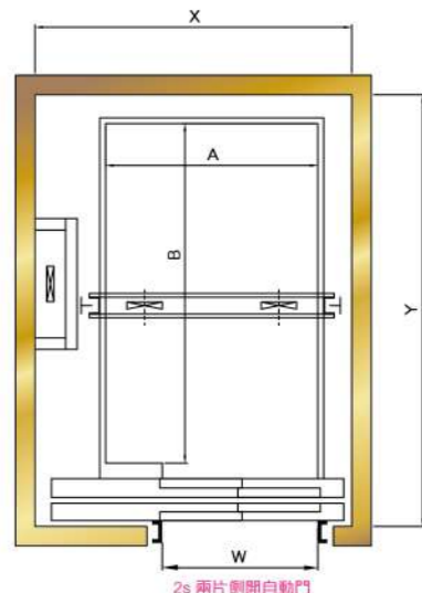
昇降道剖面圖
