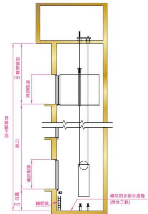
昇降道剖面圖
